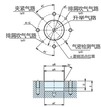
安装孔加工尺寸示意图
