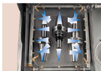
18个喷嘴自动清洗
